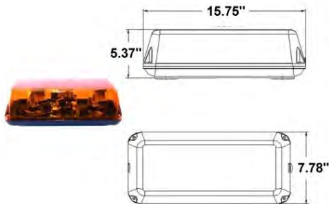
Optilux OS-400 Twin Rotating Halogen Mini Light Bar Amber Fixed Base
